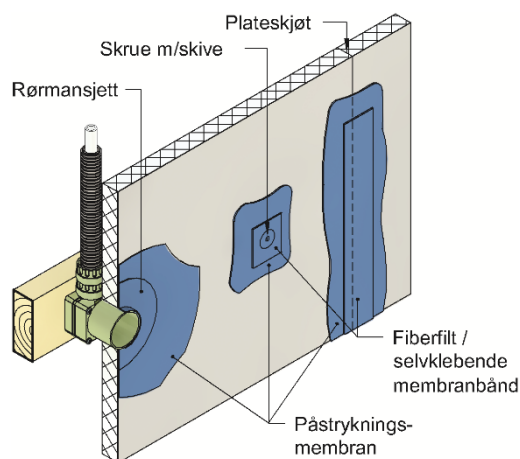
Fig. 2 Prinsipp for tetting rundt rørgjennomføringer og ved skjøter
