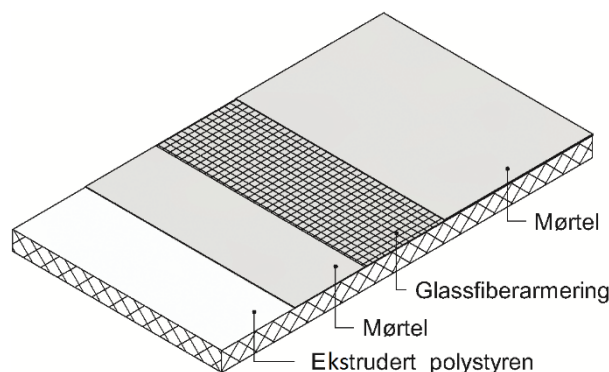
Fig. 1 Nordic Tools våtromsplate
